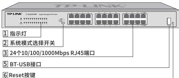
图1-3 TL-SG2024MP前面板示意图
