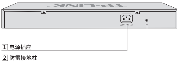
图1-5 TL-SG2226P后面板示意图
