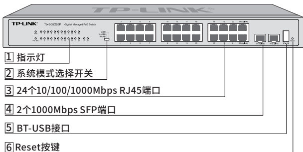
图1-2 TL-SG2226P前面板示意图
